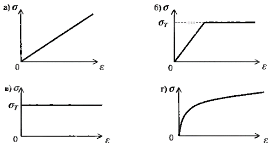
Рисунок 1 – Диаграммы деформирования материала: а – линейно-упругий; б – идеально упругопластический; в – жесткопластический; г – нелинейно упругий.
