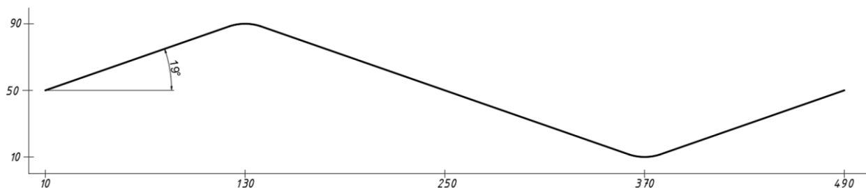
Рисунок 6 – Расположение точек ГС 480x80x6/30 по координатам (материал авторов).
