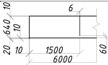
Рисунок 5 – Размеры подкрановой балки с плоской стенкой:
